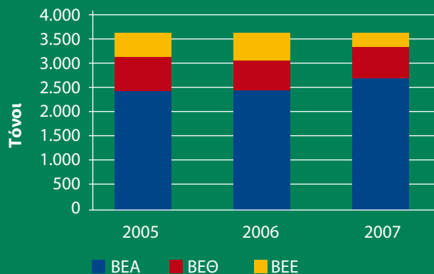
Διάγραμμα: Εκπομπές οξειδίων του αζώτου από τα διυλιστήρια Θεσσαλονίκης (BEΘ), Ασπροπύργου (BEA) και Ελευσίνας (BEE)
