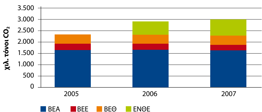
Διάγραμμα: Εκπομπές διοξειδίου του άνθρακα των Ελληνικών διυλιστηρίων του Ομίλου (BEA, BEE, BEO) και της μονάδας της θυγατρικής ΕΝΕΡΓΕΙΑΚΗ ΘΕΣΣΑΛΟΝΙΚΗΣ (ΕΝΘΕ)
