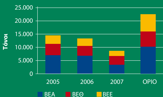
Διάγραμμα: Εκπομπές διοξειδίου του θείου από τα διυλιστήρια Θεσσαλονίκης (BEΘ), Ασπροπύργου (BEA) και Ελευσίνας (BEE)
